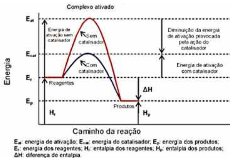
Figura 1 – Efeito do uso dos catalisadores na velocidade das reações químicas.
