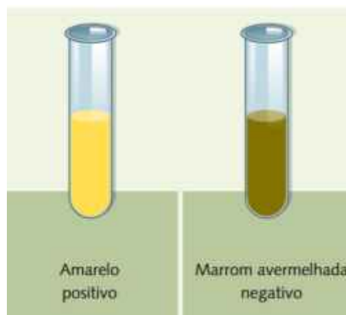
Figura 2 – resultado de análise de cloretos
