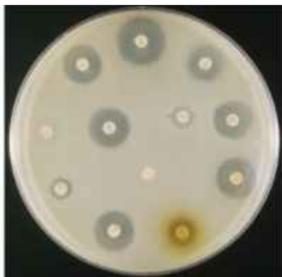
Figura 1 – Discos dispostos sobre a placa e a formação do Halo no entorno de colônias
