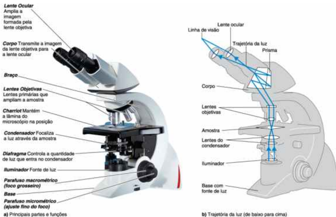
Figura 1 – Partes do Microscópio Óptico
