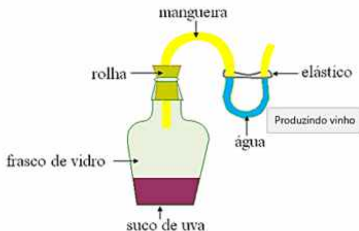
Figura 1 – Esquema da produção de vinho.
