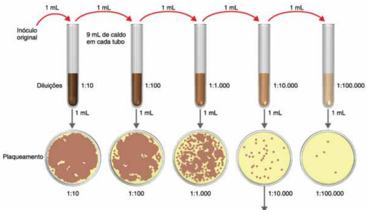
Figura 1 – Exemplo de diluição seriada e inoculação na placa de Petri correspondente.
