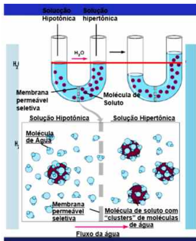
Figura 1 – Representação da Osmose. “Clusters” são aglomerados
