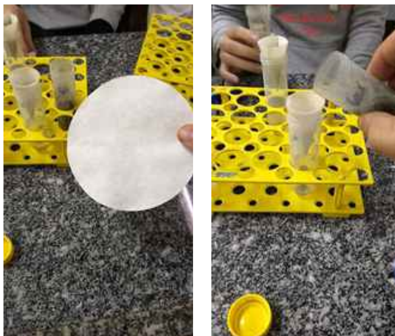
Figura 2 – Filtro de papel (à esquerda) e momento da filtração (à direita)
