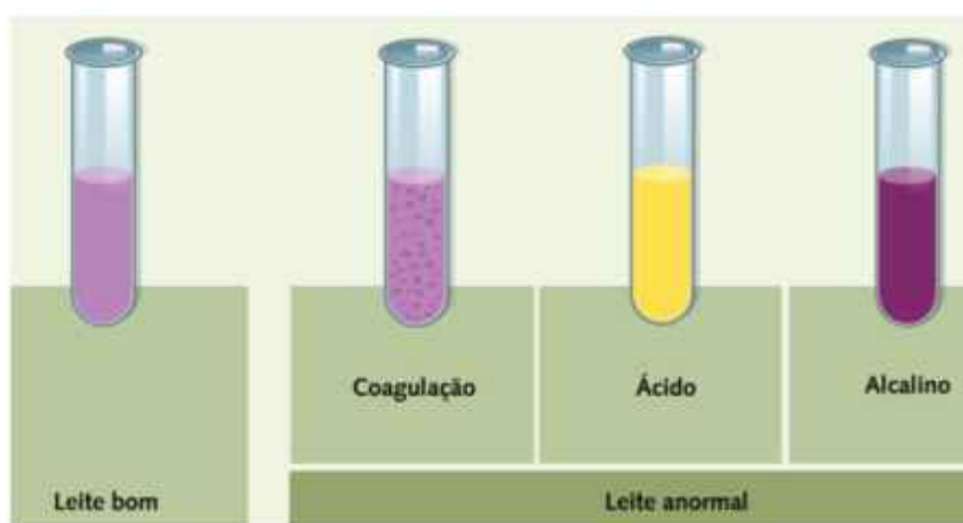
Figura 1 – Resultado da análise do Alizarol
