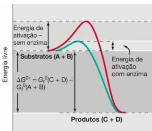
Gráfico 1 – energia de ativação e catálise.
