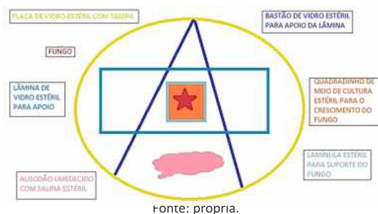
Figura 2 – Arranjo da placa de Petri para fins do microcultivo.
