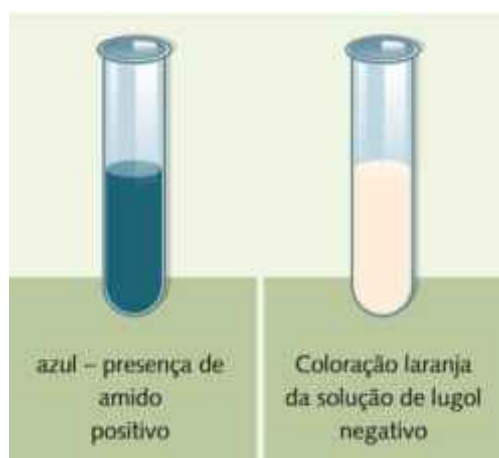
Figura 3 – Resultado para análise de amido
