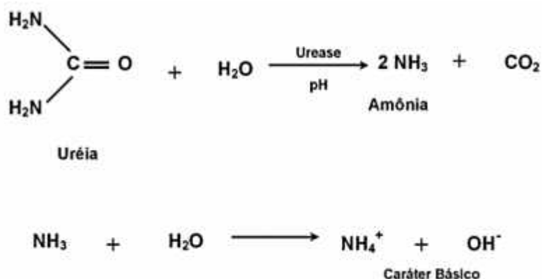
Figura 2 - Reação de decomposição da ureia e caráter básico da amônia em meio aquoso.
